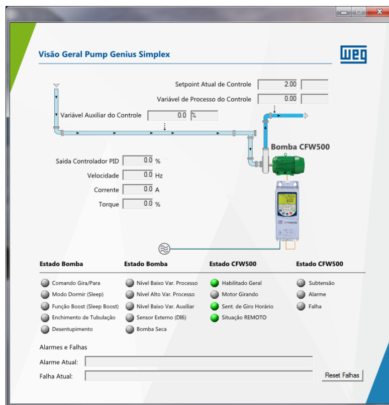
Figura 6.4 – Diálogo de monitoração da aplicação Pump Genius Simplex
