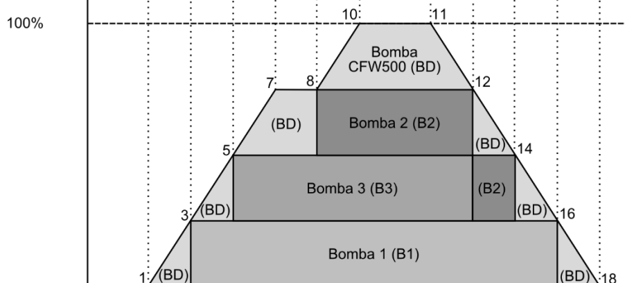
Figura 2.19 – Descritivo de funcionamento do Pump Genius configurado para controle fixo
