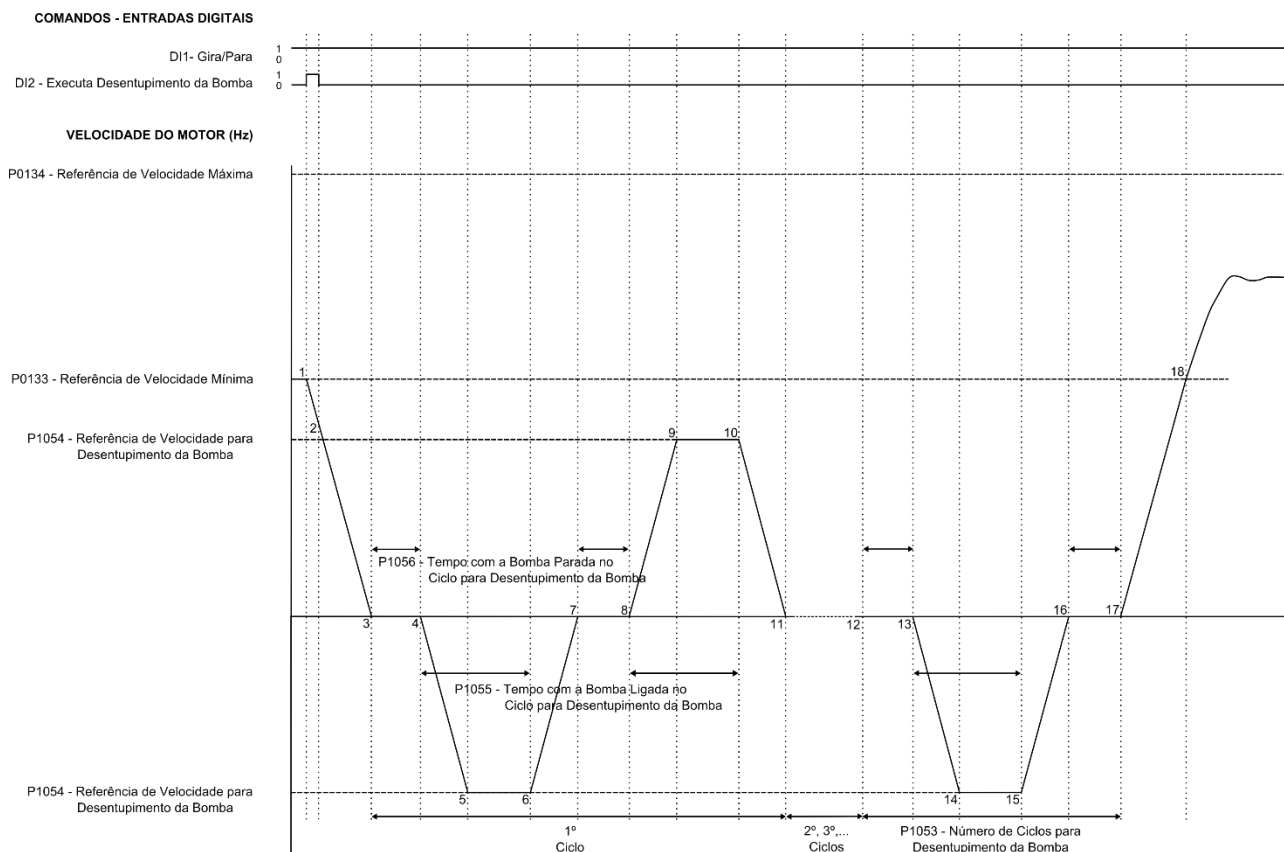
Figura 3.10 – Funcionamento do desentupimento da bomba com comando via entrada digital DI2
