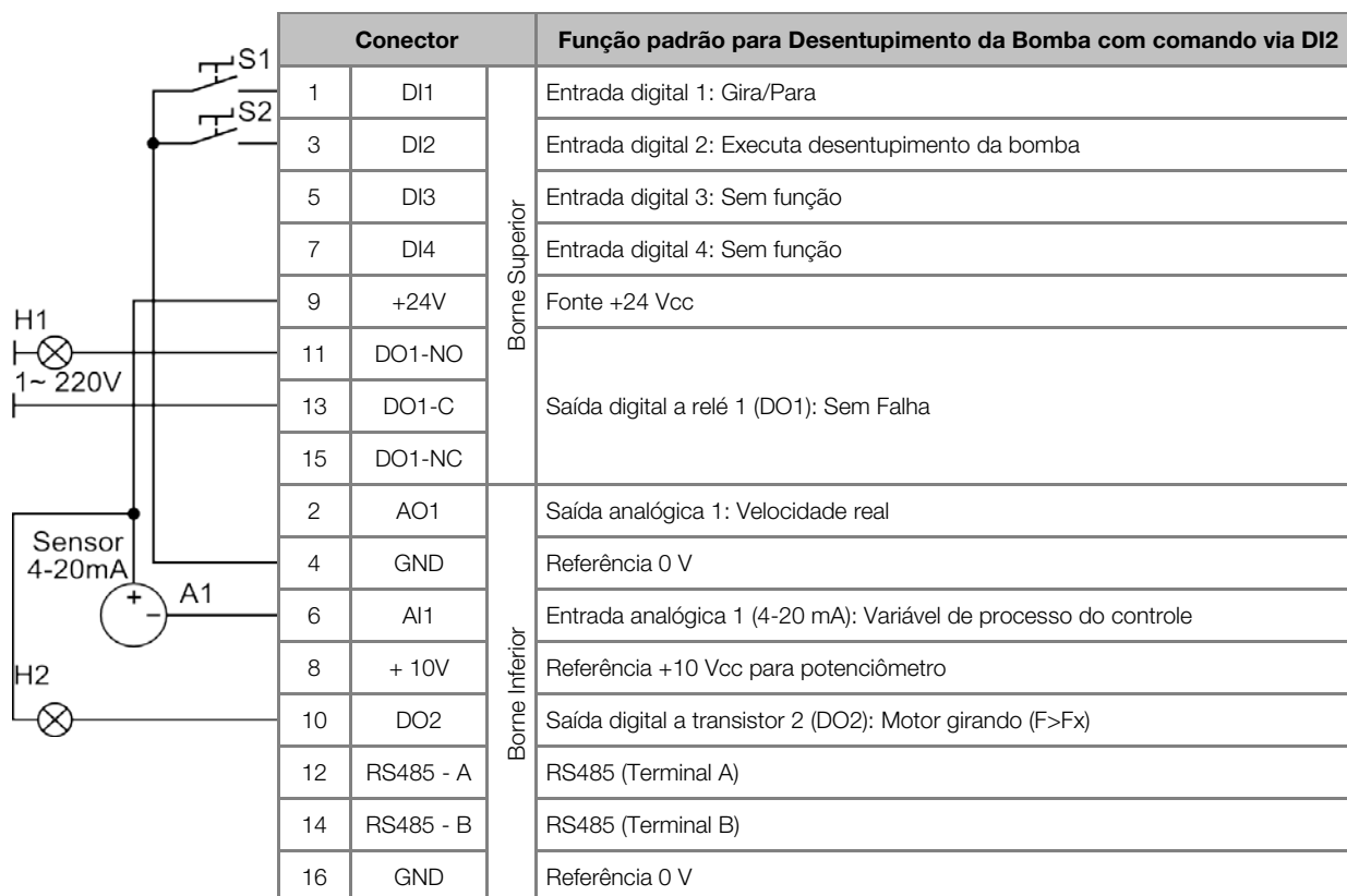
Figura 2.14 – Sinais no conector do módulo plug-in CFW500-IO5 para desentupimento da bomba com comando via entrada digital DI2
