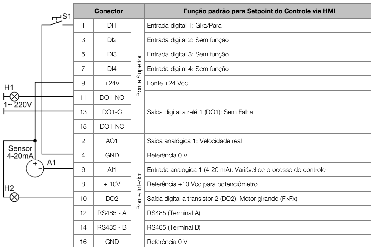
Figura 2.2 – Sinais no conector do módulo plug-in CFW500-IOS para setpoint do controle via HMI
