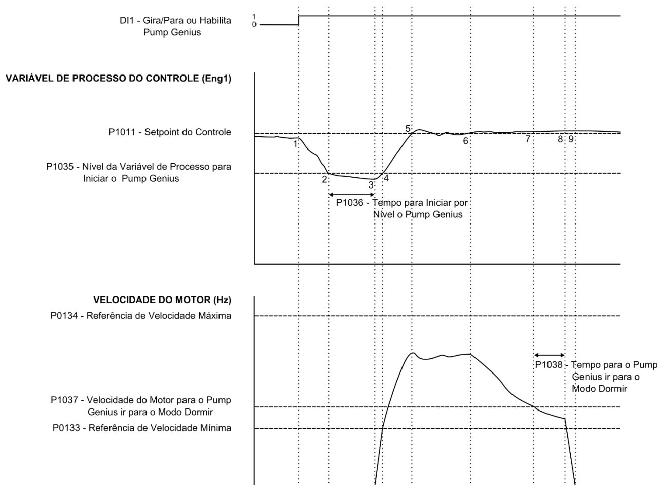
Figura 3.2 – Funcionamento do Pump Genius para modo iniciar por nível e modo dormir
