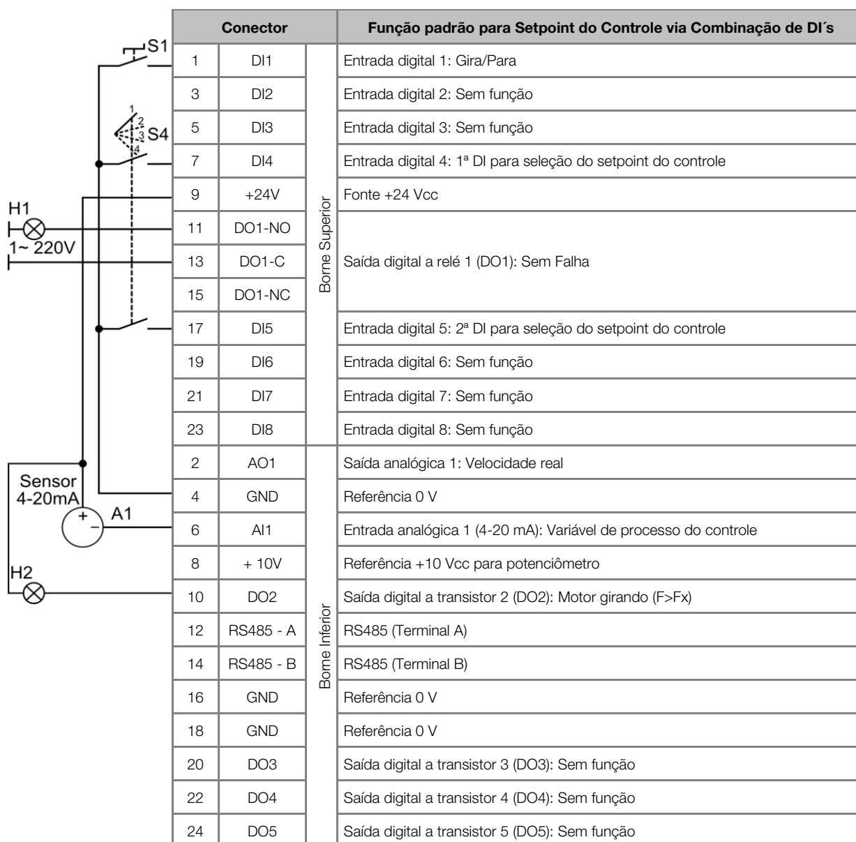
Figura 2.6 – Sinais no conector do módulo plug-in CFW500-IOD para setpoint do controle via combinação lógica das entradas digitais DI4 e DI5
