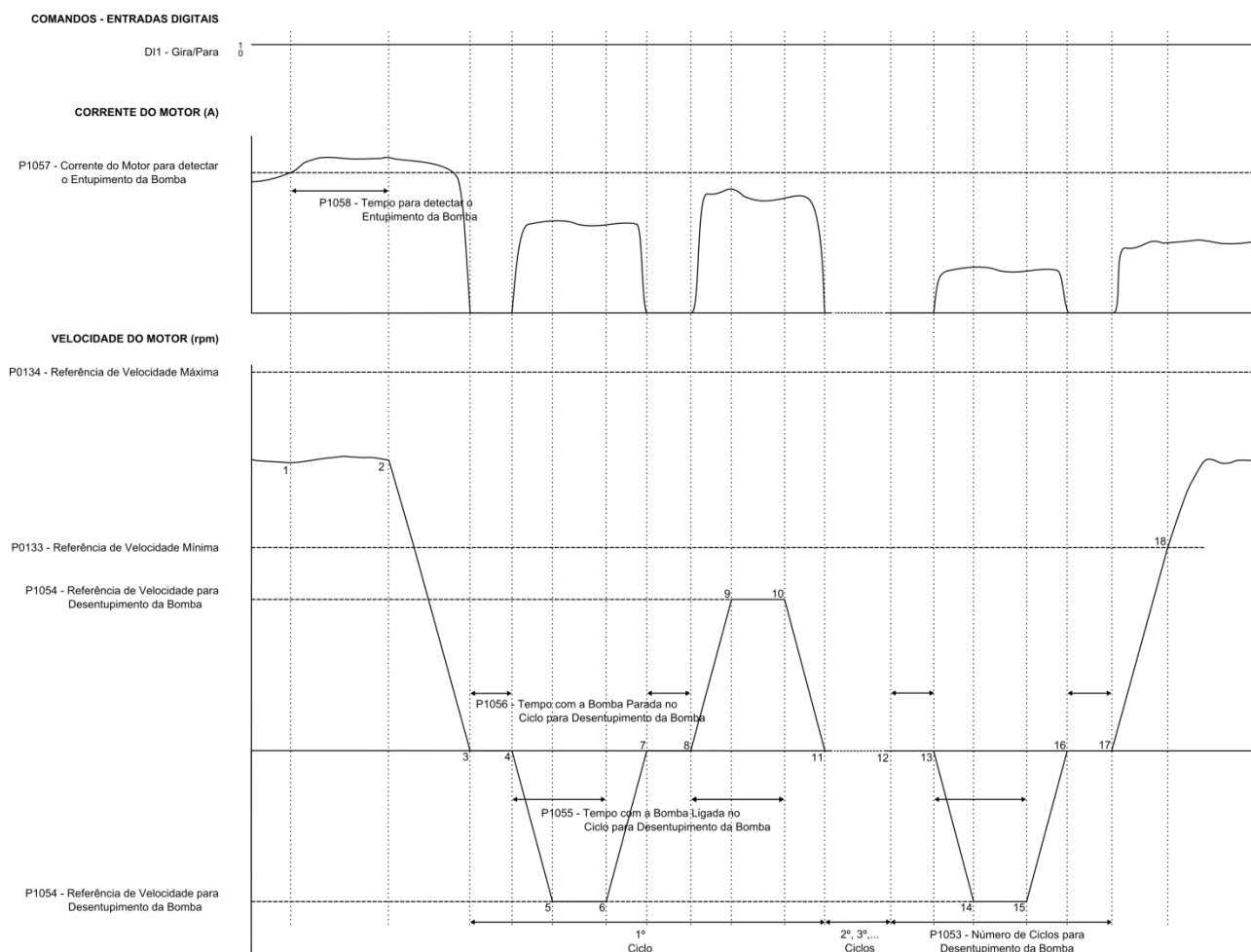
Figura 3.11 – Funcionamento do desentupimento da bomba quando detecta o entupimento da bomba
