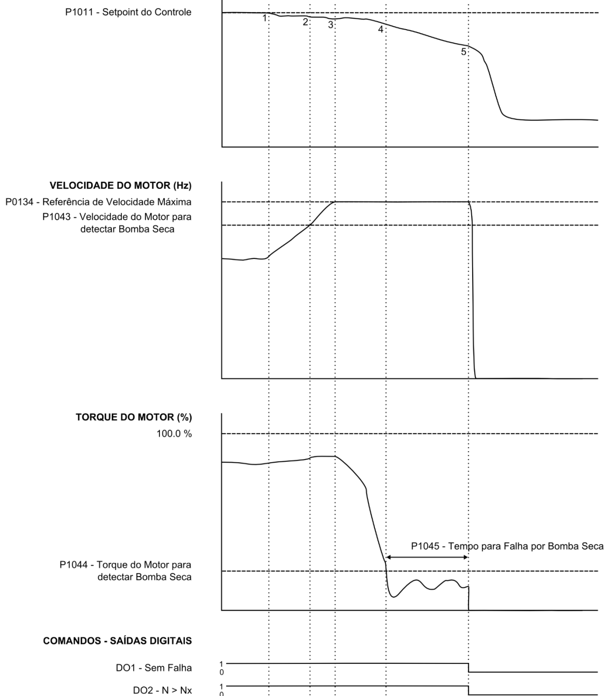
Figura 3.7 – Funcionamento do controle Pump Genius para proteção de bomba seca
