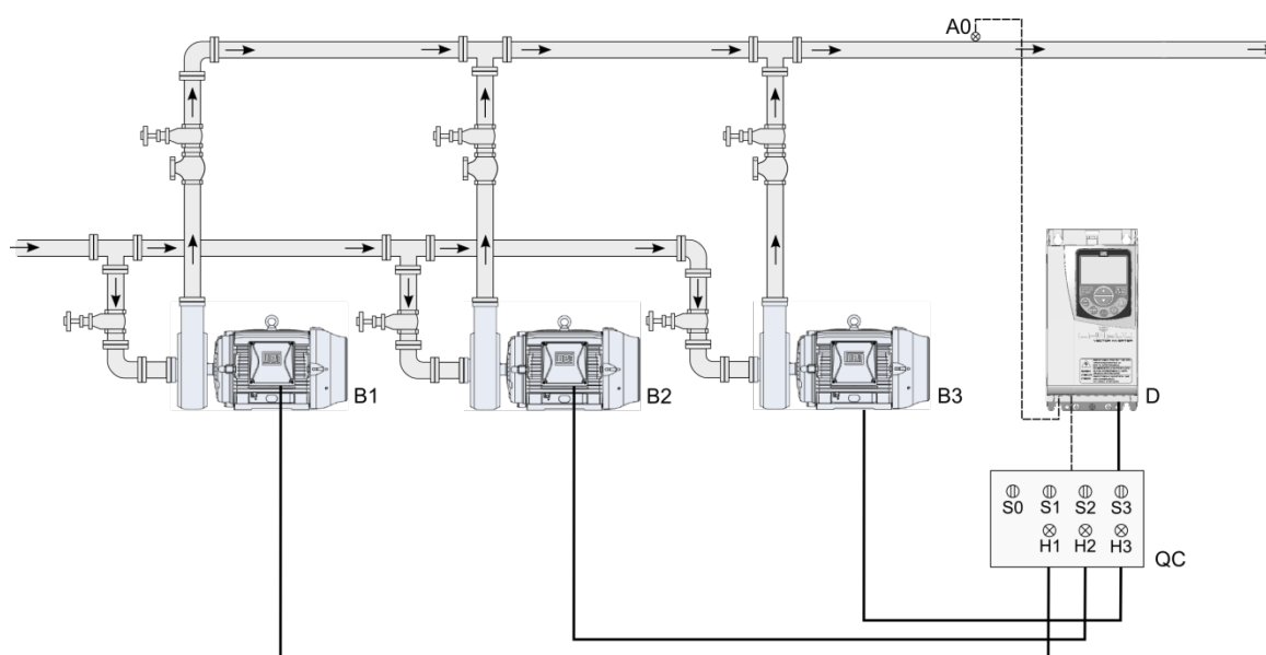
Figura 2.20 – Aplicação Pump Genius Multipump com controle móvel e três bombas em paralelo
