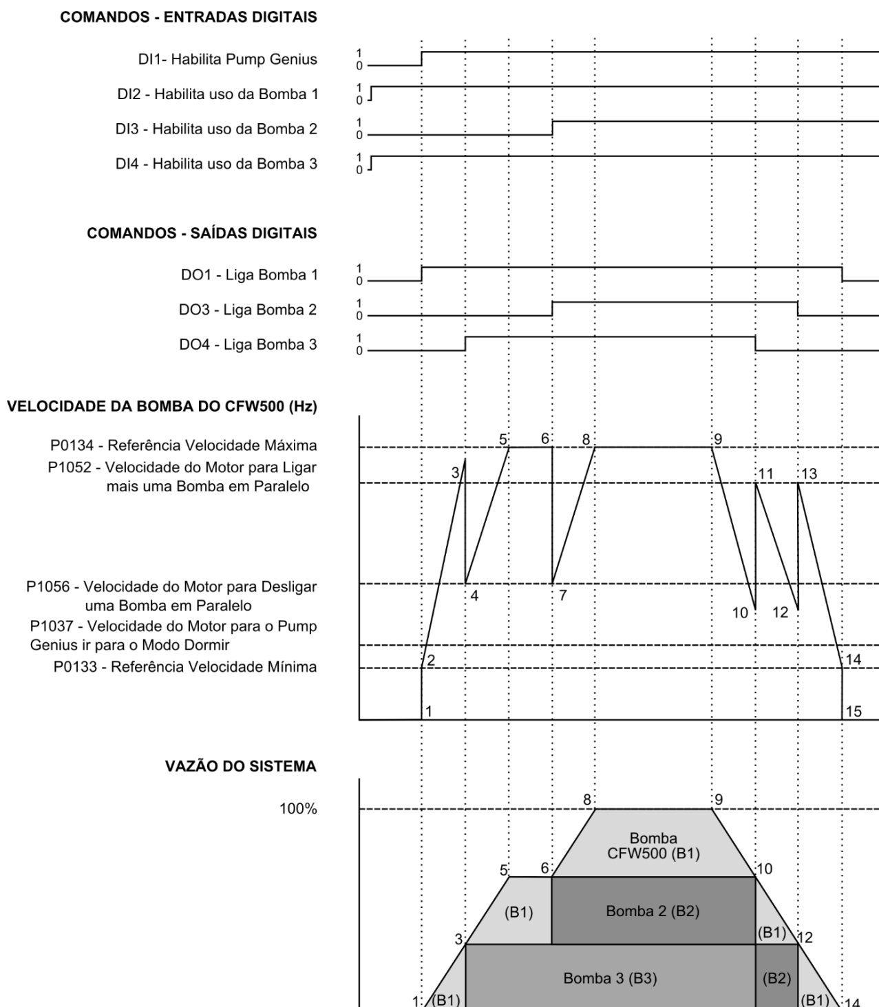
Figura 2.24 – Descritivo de funcionamento do Pump Genius configurado para controle móvel
