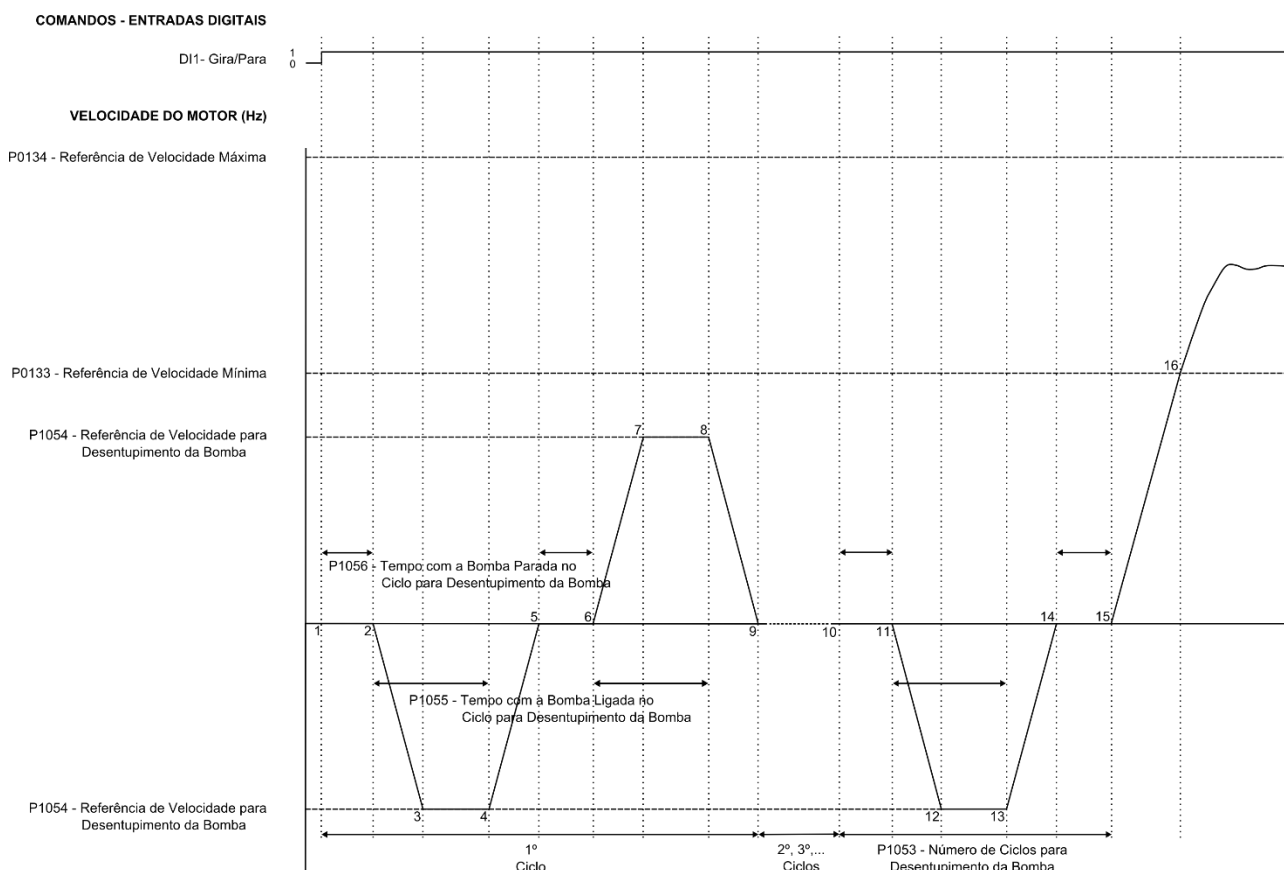
Figura 3.9 – Funcionamento do desentupimento da bomba com comando para ligar a bomba
