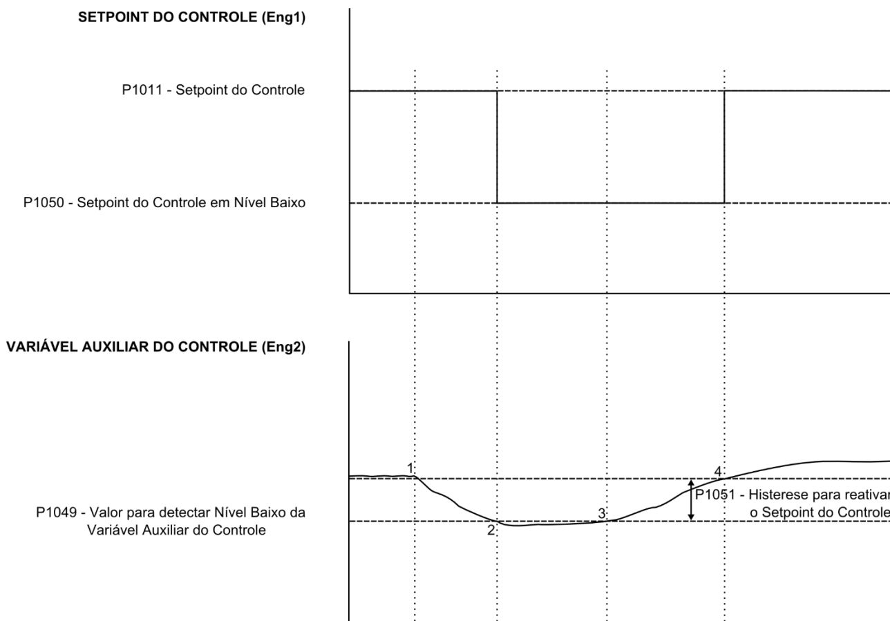
Figura 3.8 – Funcionamento do Pump Genius para proteção da bomba via variável auxiliar do controle
